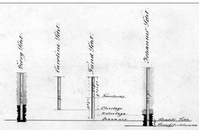
Il. 7. Profile szybów kopalni „Glückauf Ferdinand” wraz z poziomami chodników eksploatacyjnych [Ze zbioru
