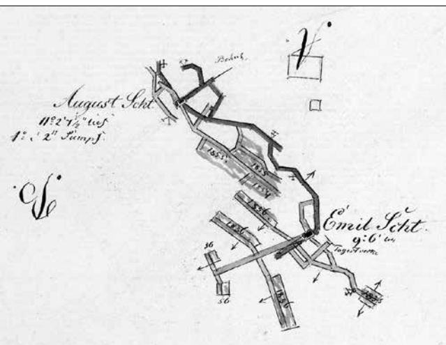
Il. 3. Fragment mapy „Grubenbild von der Glückauf Friedrich Grube bei Saabor”, 1856. Oznaczono dwa szyby
